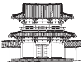
多賀城南門復元図
