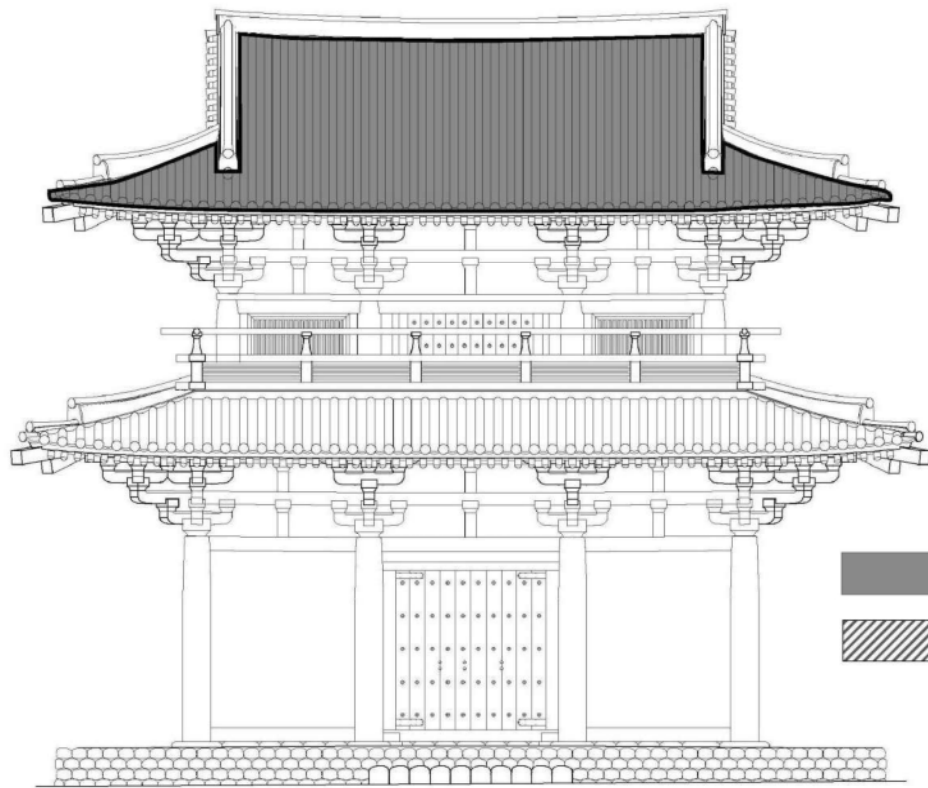
南立面図
