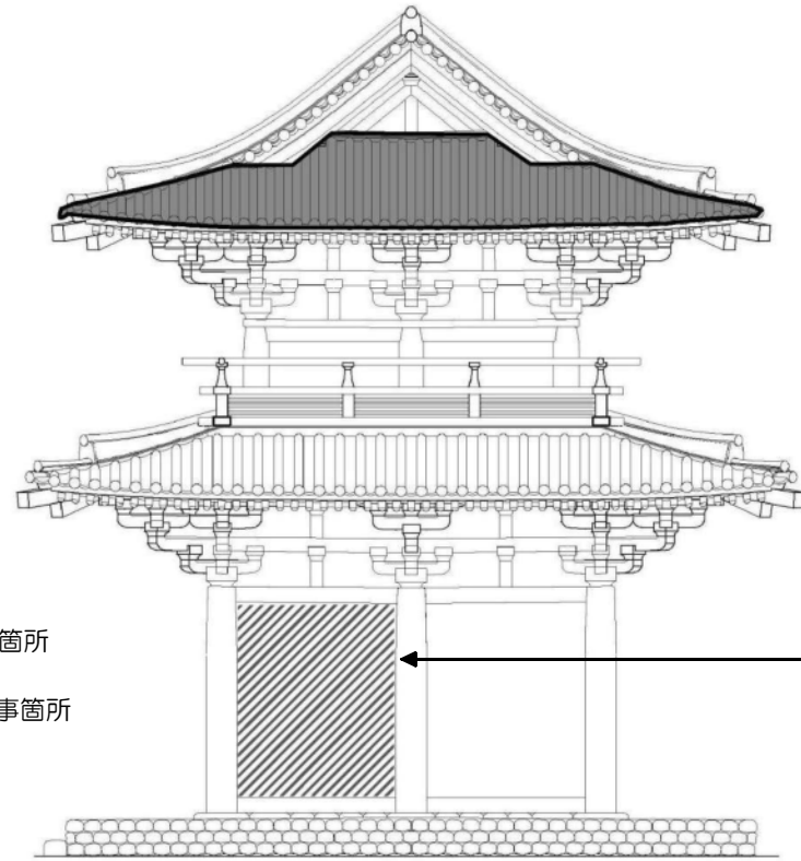
東立面図
