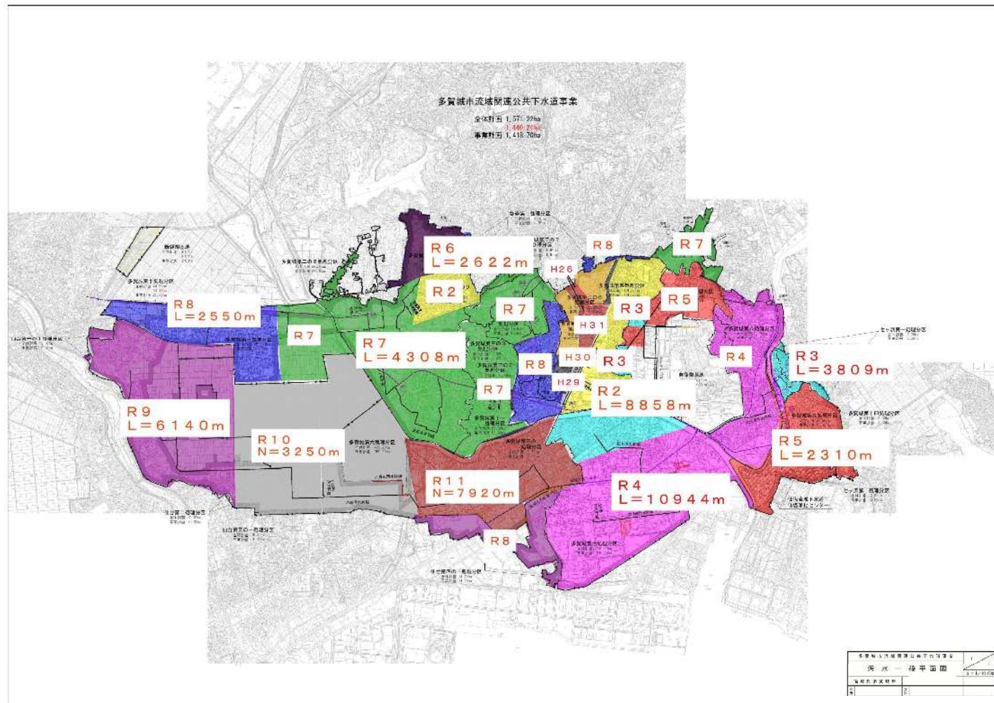
図 3.11 カメラ調査予定位置図 (管路施設)
