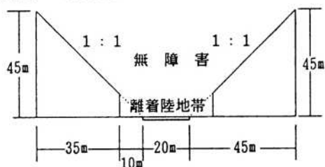
移行表面の断面図
