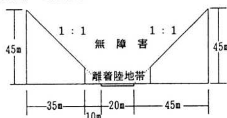
移転表面の断面図
