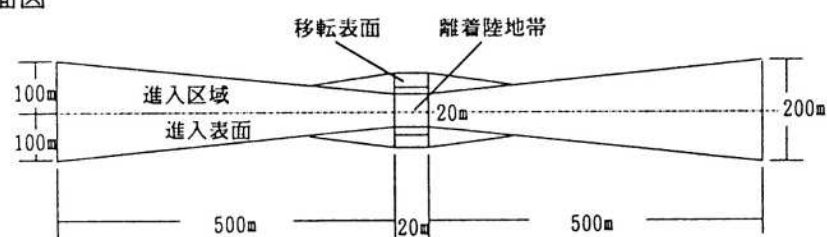
平面図
