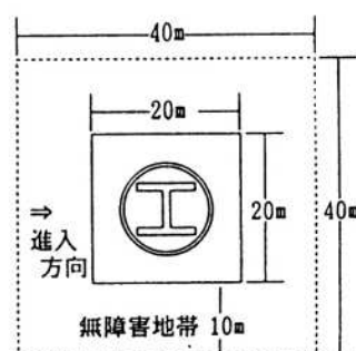
離着陸地帯平面図
