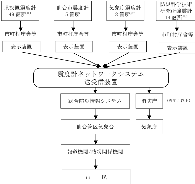
【宮城県震度情報ネットワークシステム概要図】
